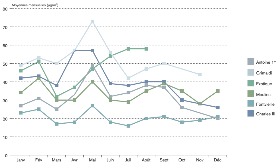
Dioxyde d'azote (NO 2 )
