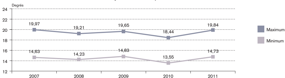
Moyenne des températures
